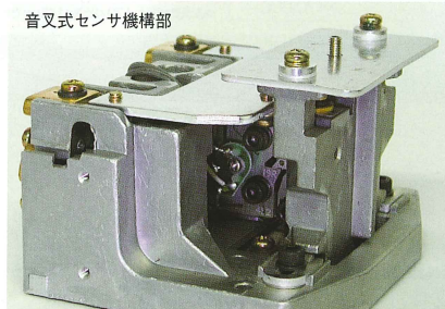
音叉式センサ機構部
