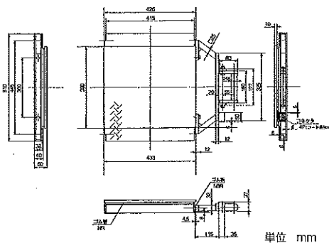
載台部図
