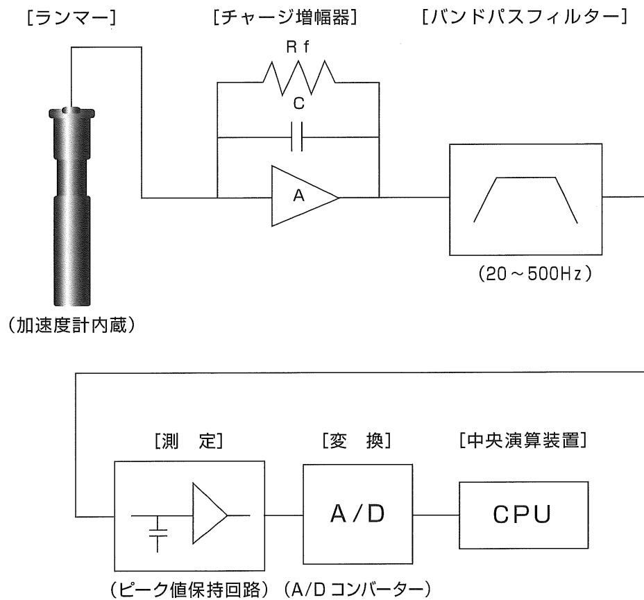
図一2 加速度計からCPUまでの回路図
