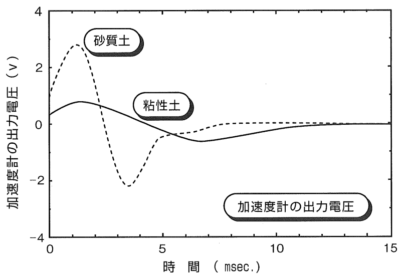
図一3 加速度計の出力波形
