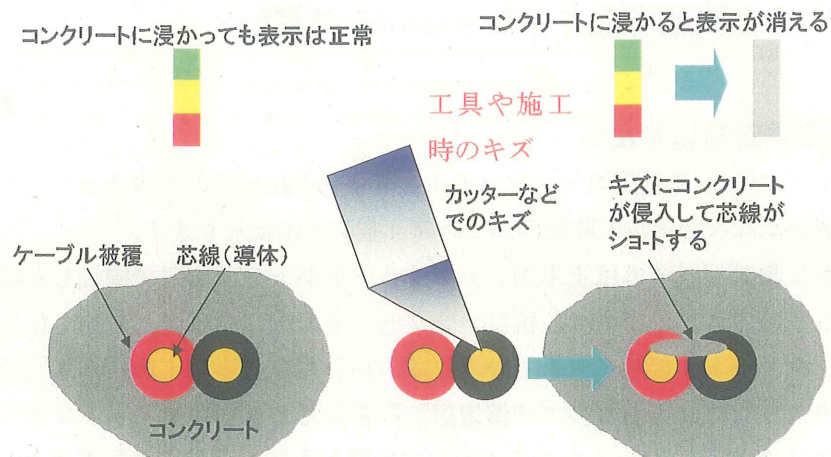
図－２ キズによるショート
