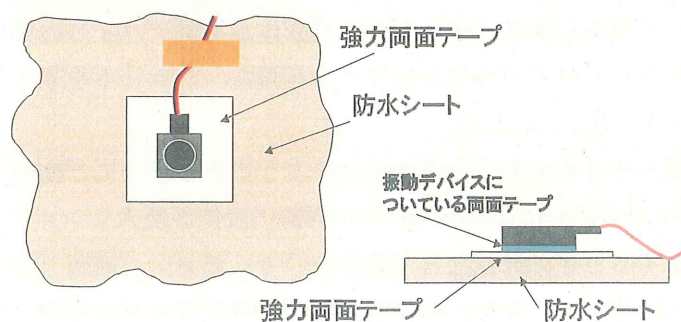
図－４ 両面テープによる下地
