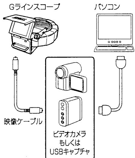
図23：接続例3
