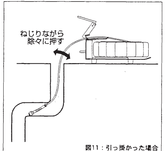
図11：引っ掛かった場合
