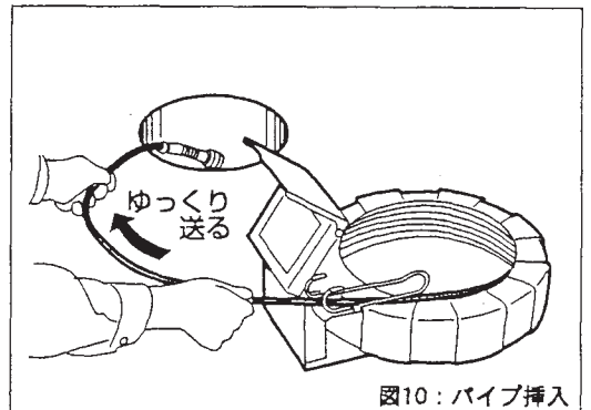
図10：パイプ挿入
