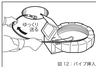
図 12：パイプ挿入
