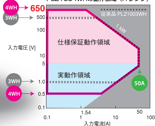
PLZ1004WHの動作領域 (Hレンジ)
