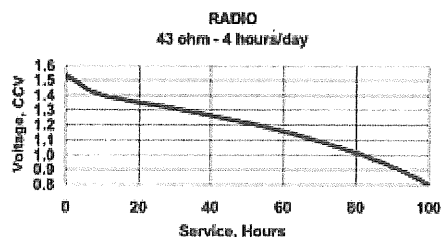
アルカリ 単三形電池 放電特性
