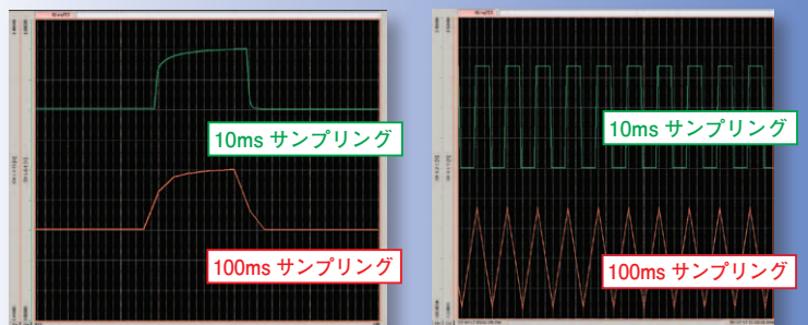
負荷が急変する波形を 10ms と 100ms でサンプリング
