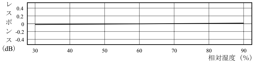
マイクロホンの湿度特性 (250 Hzにおいて)
