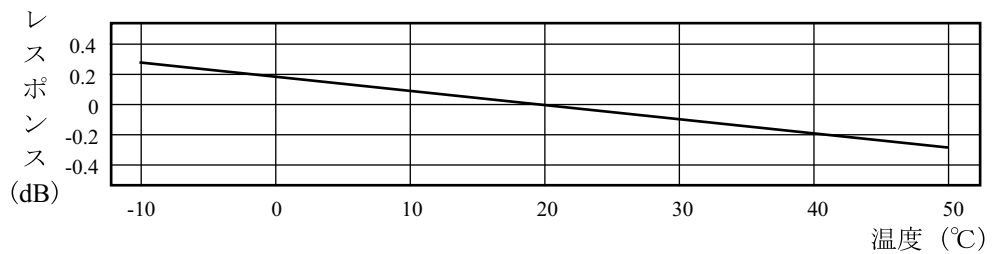
マイクロホンの温度特性 (250 Hzにおいて)
