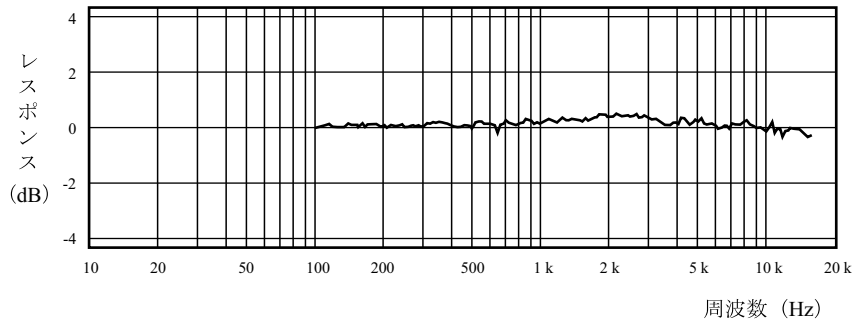
防風スクリーン WS-10 によるマイクロホンの音響的性能に対する影響（マイクロホンのみの特性を基準とする）
