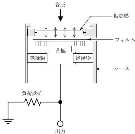
エレクトレットコンデンサマイクロホンの構造
