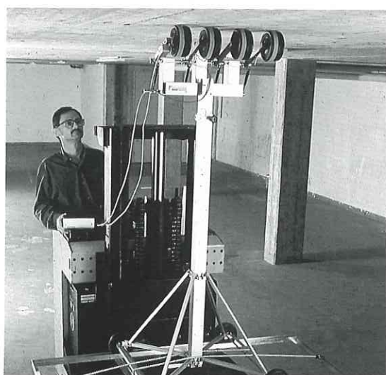
(4個のホイール電極を使用した天井面検査)
