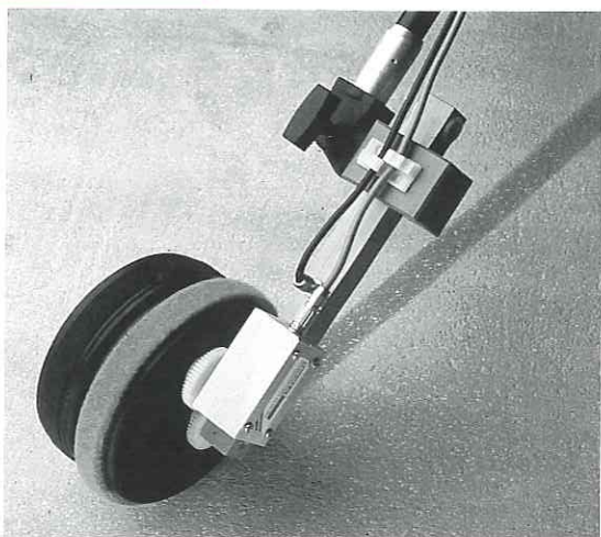
(加湿ホイール付きホイール電極)
